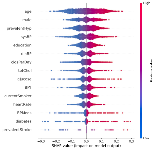
(b) SHAP
