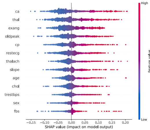
(b) SHAP
